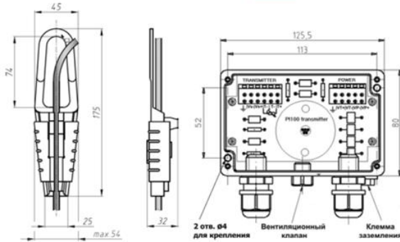
Рисунок 2. Установочные принадлежности.
