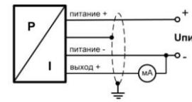
3-проводная линия (вых. сигнал - ток)
