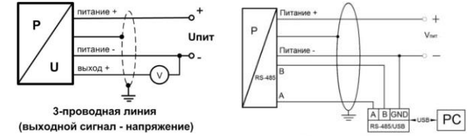
3-проводная линия (выходной сигнал - напряжение)
