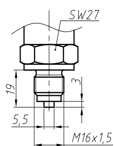
M16x1,5 EN 837
