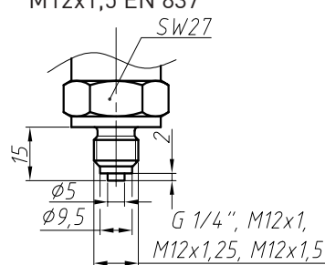
G1/4"; M12x1; M12x1,25; M12x1,5 EN 837
