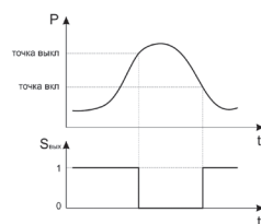
B - режим гистерезиса инверсный
