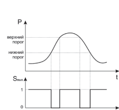
D - режим окна инверсный
