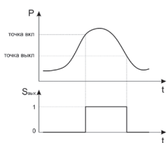
A - режим гистерезиса
