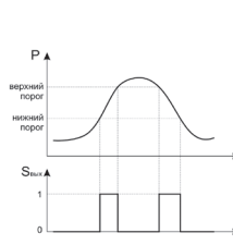
C - режим окна
