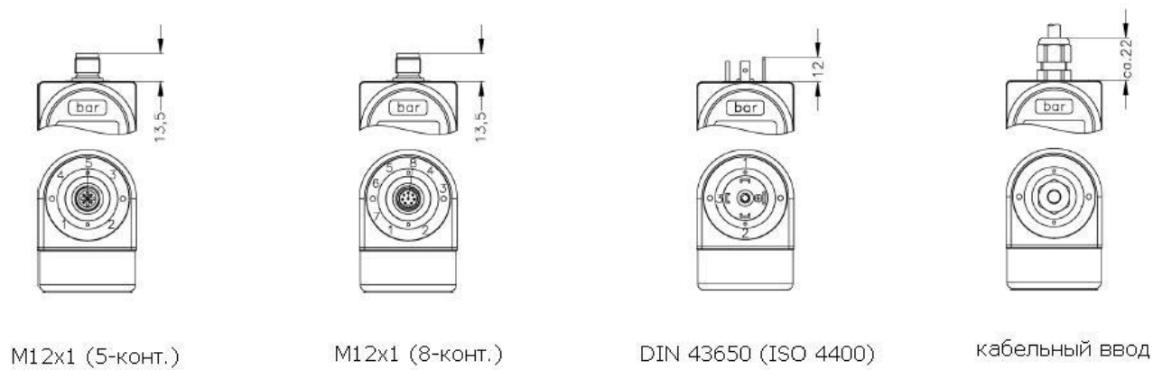
Рисунок Б.3. Типы электрических присоединений.
