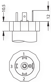
DIN 43650
