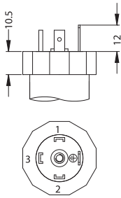
DIN 43650
